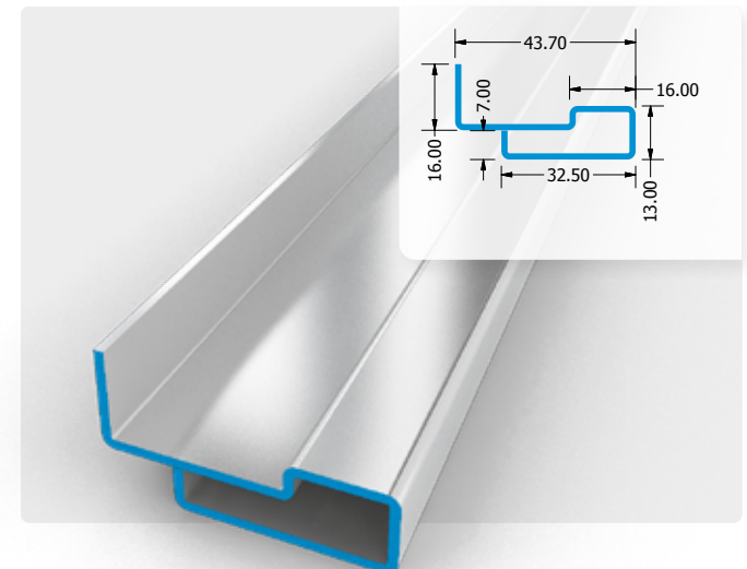
Veka 113.312
